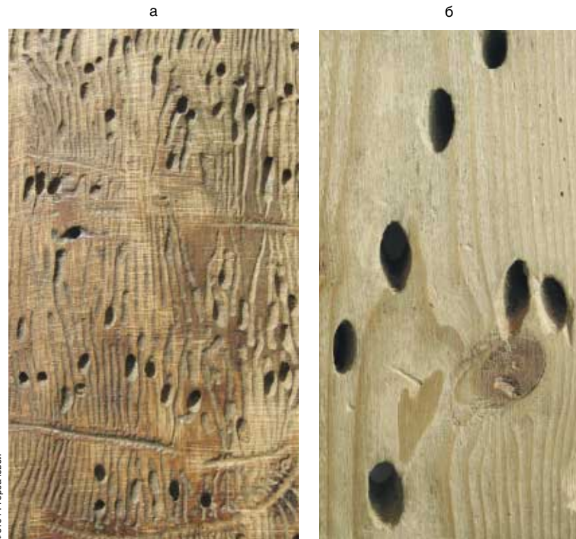
Рис. 31. Червоточина: а — поверхностная; б — глубокая в пилопродукции
