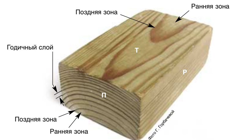
Рис. 3. Вид годичных слоев на главных разрезах
