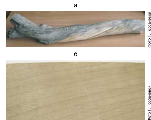
Рис. 17. Наклон волокон: а — тангенциальный наклон в круглом лесоматериале; б — радиальный наклон волокон в пилопродукции
