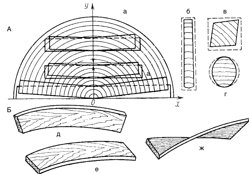
Рис. 32. Виды покоробленности:
