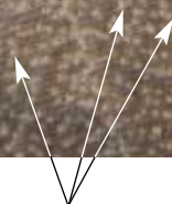
Сосуды
