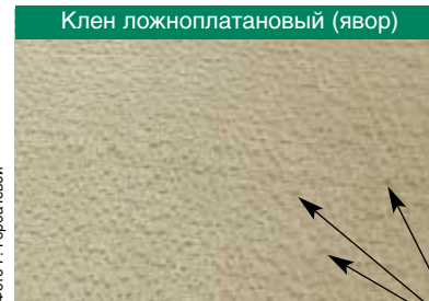
Сердцевинные лучи
